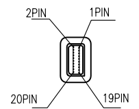
Conn.1 Mini Display Port
